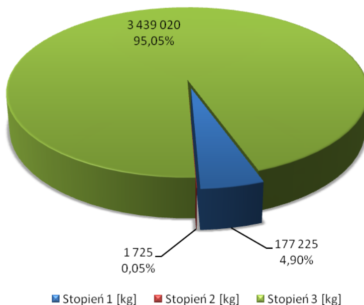
Rysunek 7. Ilość wyrobów zawierających azbest w procentowym podziale na stopnie pilności usunięcia w Gminie Korczew.
