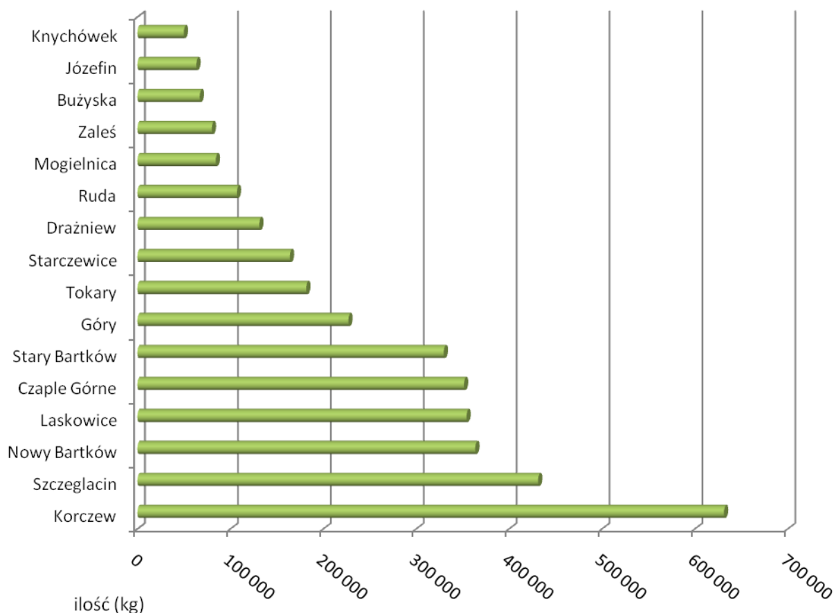
Rysunek 6. Porównanie ilości zinwentaryzowanych wyrobów zawierających azbest dla poszczególnych obrębów ewidencyjnych Gminy Korczew (kg).
